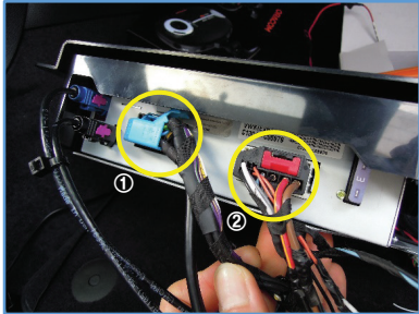
보조석 시트 밑 'EX-BOX' 본체 뒷 면
