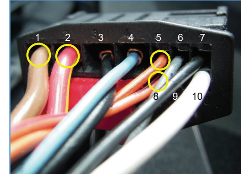
10핀 커넥터 (2) 배선 정보
