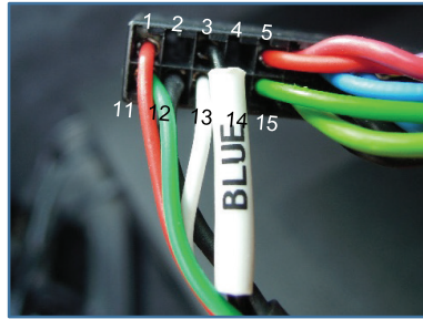
RGB 배선 터미널(5개)을 각 핀 위치에 삽입
