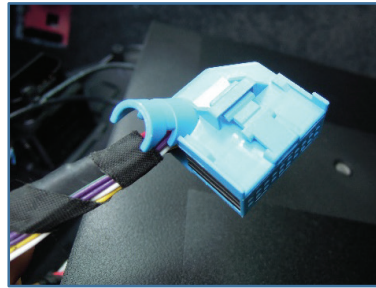
20핀 커넥터(1) 분리 후, 하네스 제거
