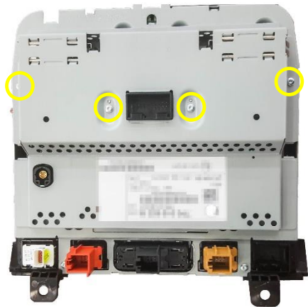
※ 스크류 제거후 모니터 커버 분리
