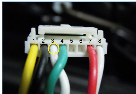
3) 54핀 커넥터의 '1번 핀(노란색/적색) 배선'에 모듈 커넥터 '3번 핀(흰색) 배선'을 연결 < CAN HIGH 연결 >
