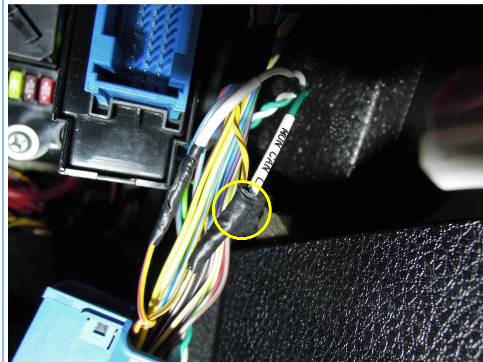
4) 54핀 커넥터의 '2번 핀(노란색/갈색) 배선'에 모듈 커넥터 '4번 핀(녹색) 배선'을 연결 < CAN LOW 연결 >
