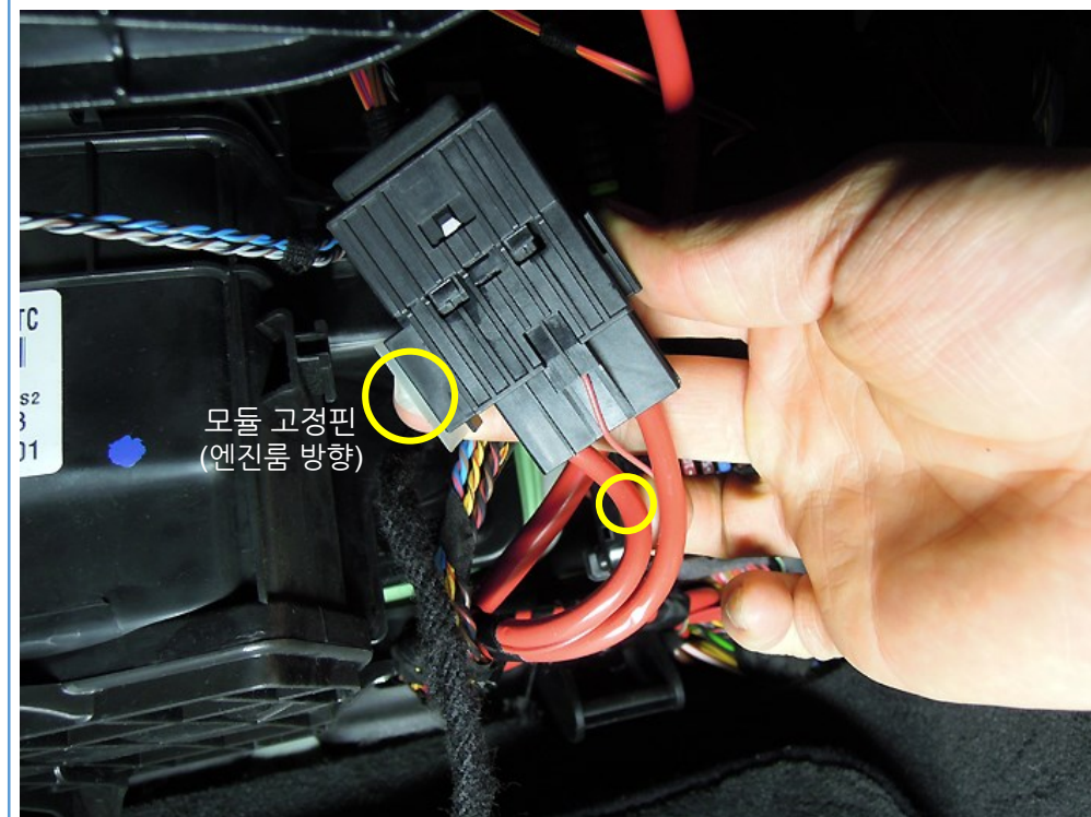
6) '엔진룸 방향'의 '굵은 적색 배선(배터리 전원)'에 모듈 커넥터 '1번 핀(노란색) 배선'을 연결 < 전원 연결 > / 2번 배선(GROUND) 차량의 접지와 연결
