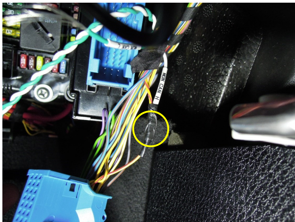
3) 54핀 커넥터의 '1번 핀(노란색/적색) 배선'에 모듈 커넥터 '3번 핀(흰색) 배선'을 연결 < CAN HIGH 연결 >
