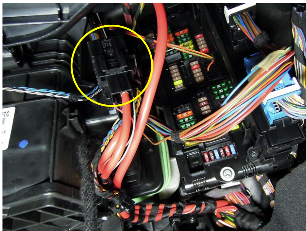
5) 휴즈박스 앞, 표시된 '릴레이 모듈'을 시계 반대 방향으로 돌려 분리
