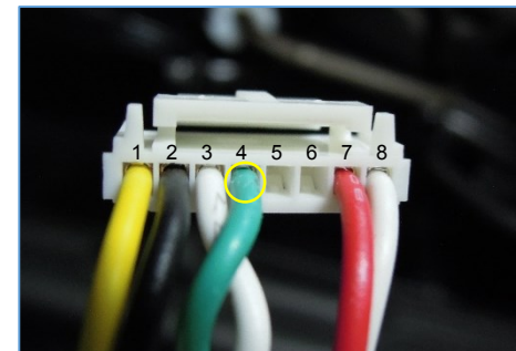
4) 54핀 커넥터의 '2번 핀(노란색/갈색) 배선'에 모듈 커넥터 '4번 핀(녹색) 배선'을 연결 < CAN LOW 연결 >
