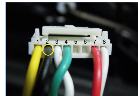
6) 모니터 커넥터의 '3번 핀(갈색) 배선'에 모듈 커넥터 '2번 핀(검정색) 배선'을 연결 < GROUND 연결 >
