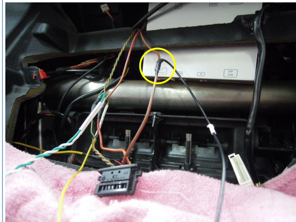
6) 모니터 커넥터의 '3번 핀(갈색) 배선'에 모듈 커넥터 '2번 핀(검정색) 배선'을 연결 < GROUND 연결 >
