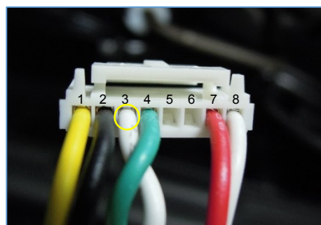
3) 모니터 커넥터의 '5번 핀(연두색/주황색) 배선'에 모듈 커넥터 '3번 핀(흰색) 배선'을 연결 < CAN HIGH 연결 >
