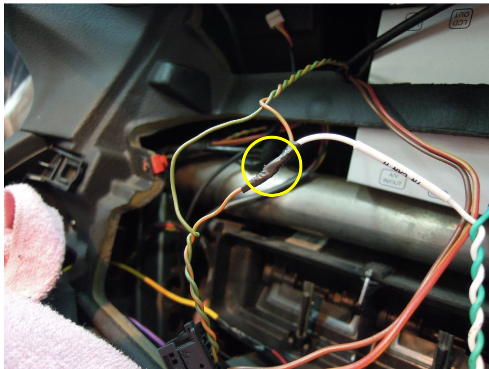
3) 모니터 커넥터의 '5번 핀(연두색/주황색) 배선'에 모듈 커넥터 '3번 핀(흰색) 배선'을 연결 < CAN HIGH 연결 >
