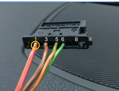
5) 모니터 커넥터의 '1번 핀(적색/노란색) 배선'에 모듈 커넥터 '1번 핀(노란색) 배선'을 연결 < 전원 연결 >
