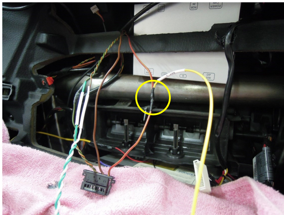
5) 모니터 커넥터의 '1번 핀(적색/노란색) 배선'에 모듈 커넥터 '1번 핀(노란색) 배선'을 연결 < 전원 연결 >
