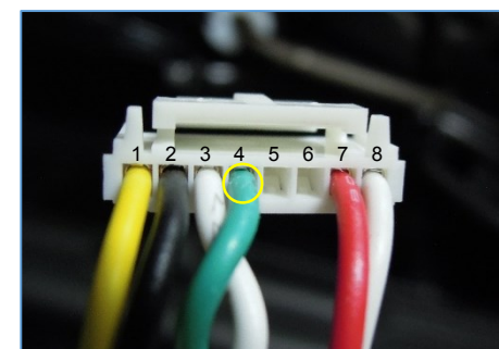
4) 모니터 커넥터의 '6번 핀(연두색) 배선'에 모듈 커넥터 '4번 핀(녹색) 배선'을 연결 < CAN LOW 연결 >
