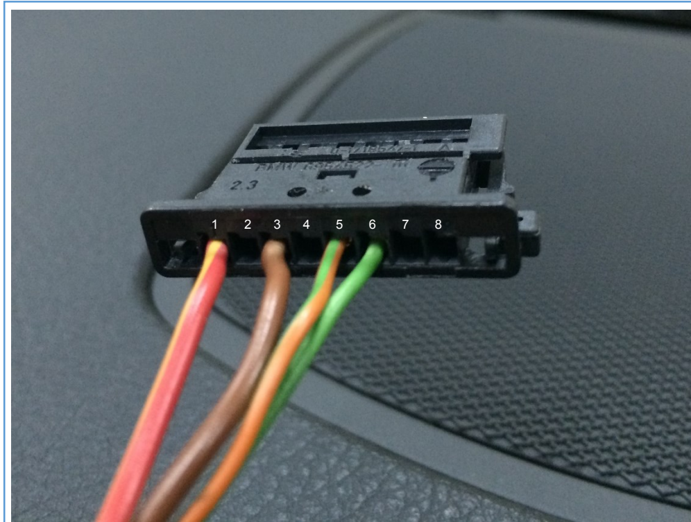
2) 모니터 8핀 커넥터 핀 사양 안내
