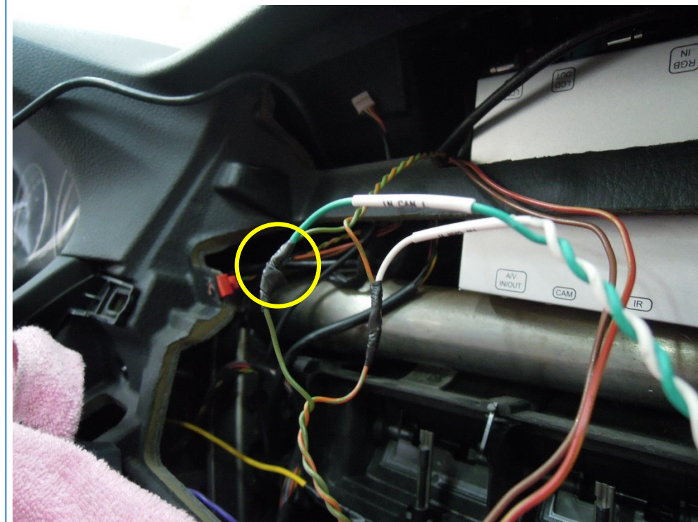
4) 모니터 커넥터의 '6번 핀(연두색) 배선'에 모듈 커넥터 '4번 핀(녹색) 배선'을 연결 < CAN LOW 연결 >
