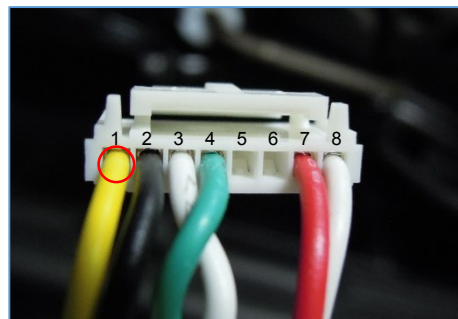
5) 모니터 커넥터의 '1번 핀(적색/노란색) 배선'에 모듈 커넥터 '1번 핀(노란색) 배선'을 연결 < 전원 연결 >
