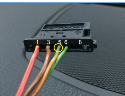
3) 모니터 커넥터의 '5번 핀(연두색/주황색) 배선'에 모듈 커넥터 '3번 핀(흰색) 배선'을 연결 < CAN HIGH 연결 >
