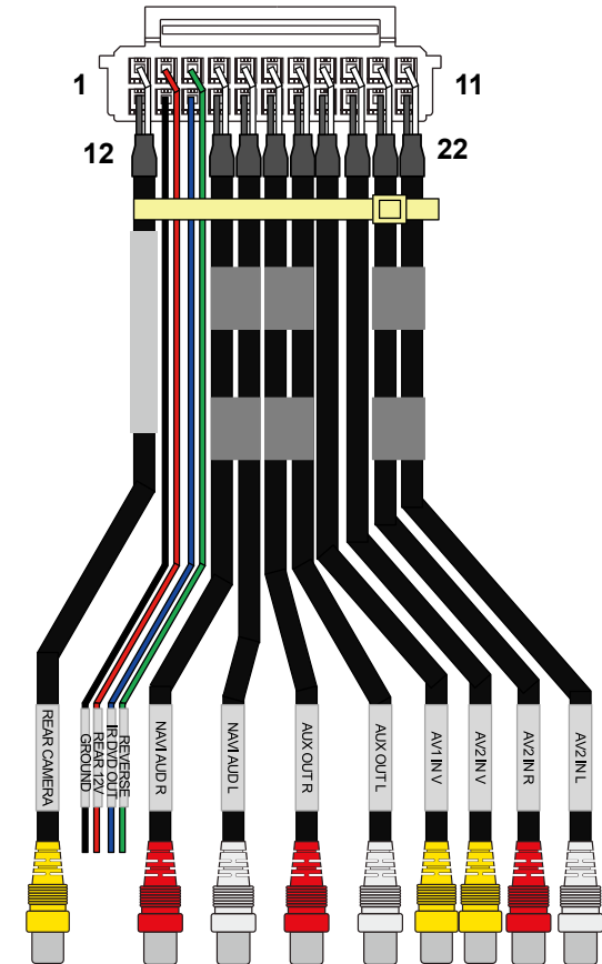
AV CABLE
