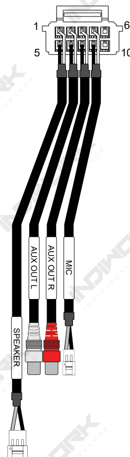
AV Cable
